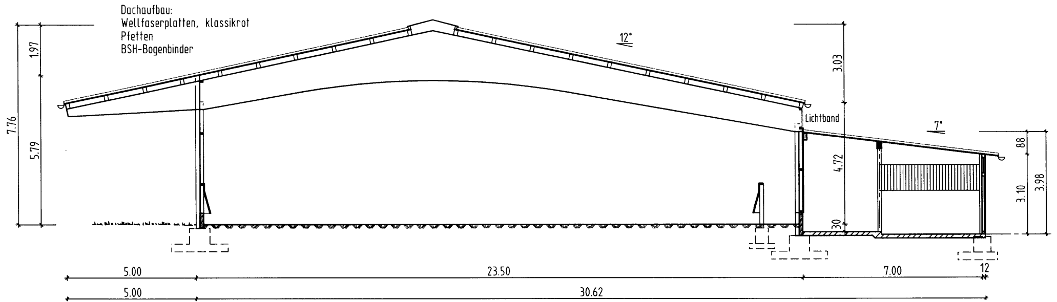
Schnitt A-A
